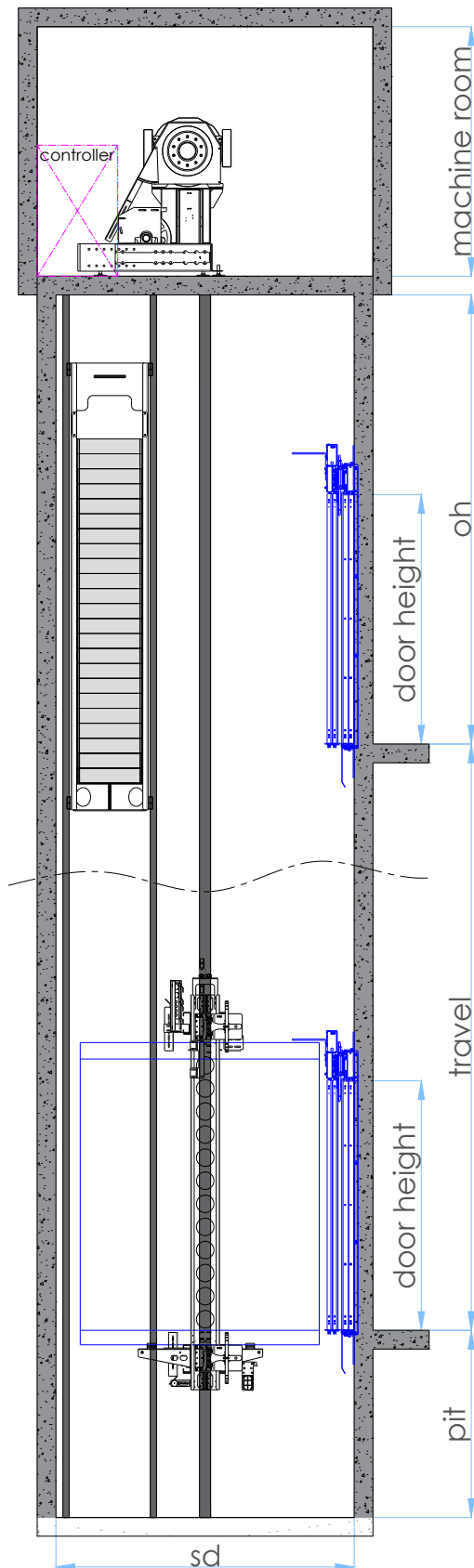
SECTION A-A
